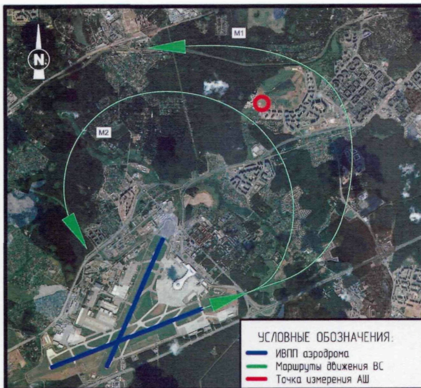
Рис. 7. Схема расположения точки (места) измерения относительно маршрутов взлета с МК=058° аэродрома
