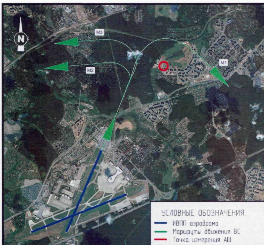
Рис. 8. Схема расположения точки (места) измерения относительно маршрутов взлета с МК=013° аэродрома
