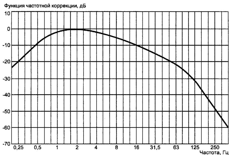
Рисунок А.1 - Функция частотной коррекции W_m для сигнала ускорения
