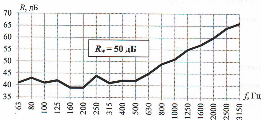
Частотная характеристика звукоизоляции
